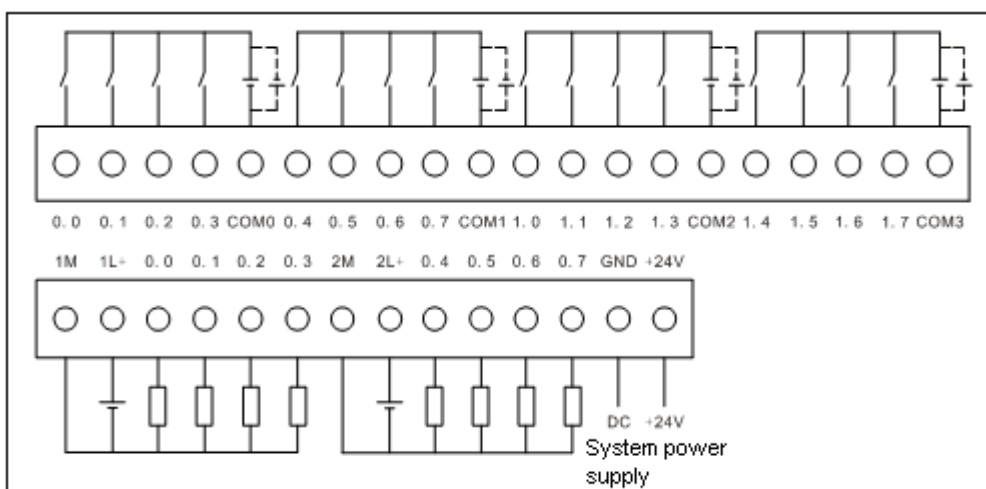
Рис. 2.5 Схема подключения цифровых входов/выходов RP2D-1608C1
